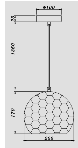
DIMENSIONS
