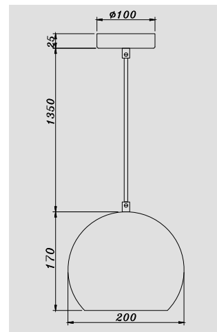
DIMENSIONS
