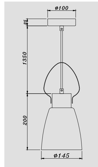
DIMENSIONS
