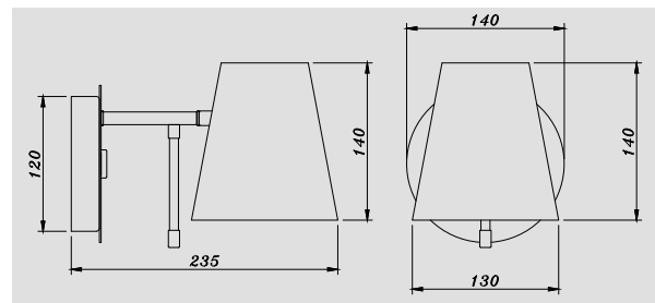
DIMENSIONS
