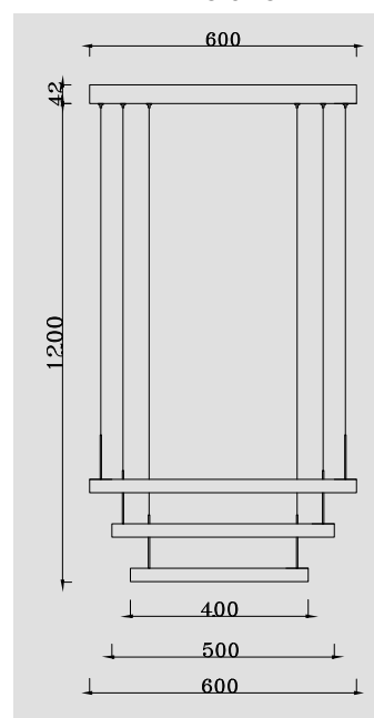
DIMENSIONS
