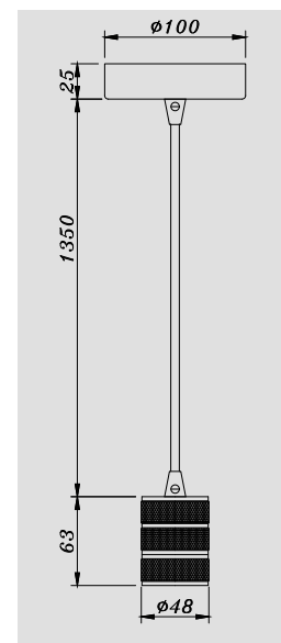
DIMENSIONS
