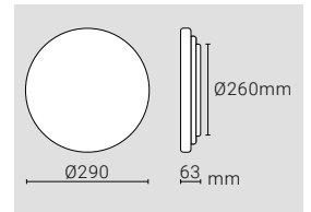
20W - DIMENSIONS
