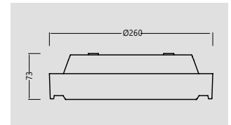
DIMENSIONS - 13W
