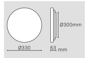
24W - DIMENSIONS
