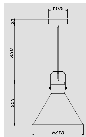
DIMENSIONS
