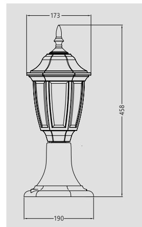
DIMENSIONS
