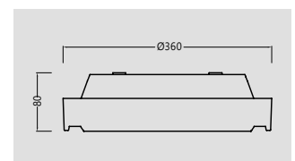
DIMENSIONS - 20W
