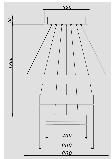
DIMENSIONS
