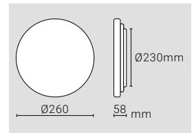
14W - DIMENSIONS
